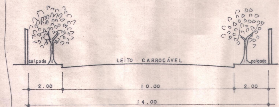
CORTE TRANSVERSAL DAS RUAS ESC. 1:125
