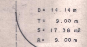
DETALHE CURVA ESQUINA ESC. 1:500
